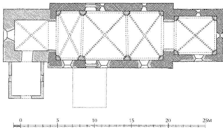
Fig. 5. Grundplan. 1:300. Tegnet af Merete Rude 2012 efter opmåling af arkitektfirmaet Birch & Svenning 2007, suppleret af NJP. – Grund plan.
