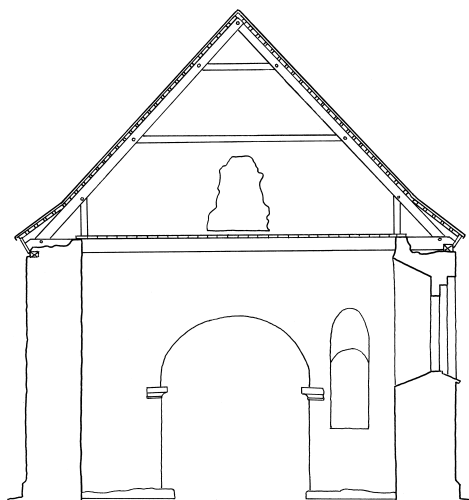
Fig. 6. Tværsnit 1:150 gennem skibet set mod øst. Målt og tegnet af Peter Duun 2009. – Querschnitt durch Schiff gegen Osten.
