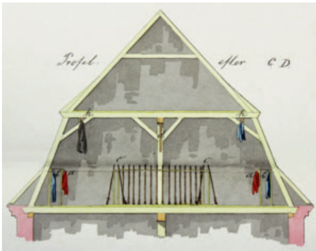
Plan for nyindretning af et munderingskammer i Glückstad 1838. Tegningen giver et glimrende indtryk af de munderingskamre, som fandtes i alle danske og slesvig-holstenske garnisonsbyer. Rigsarkivet.
